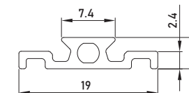
C槽专用铝杆
