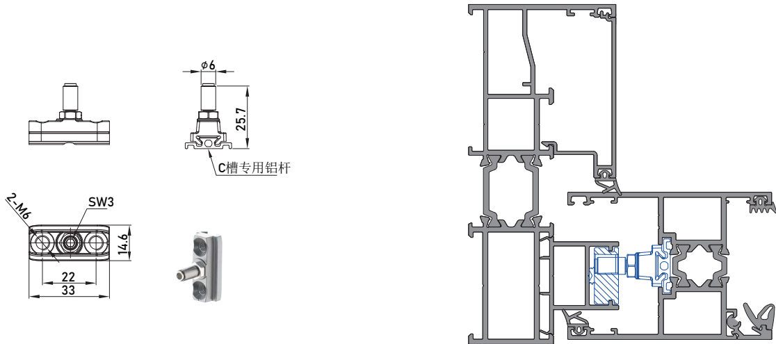
20槽侧压锁点 零件编号:K00967
