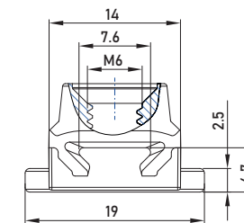
C槽专用接驳头
