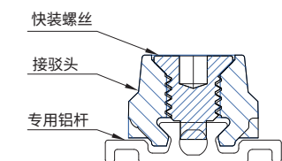
连接示意图
