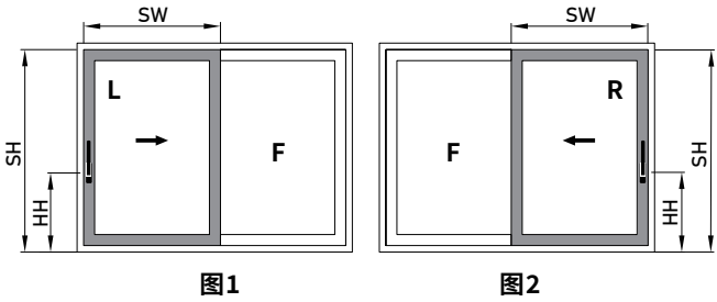
图1: 宝高标准，左开，左扇执手 GB/T 5823 右推拉门（室外侧） DIN EN 12519 右推拉（right opening）
