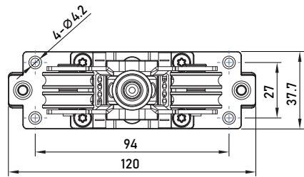
W3730双排侧压下轮 编号:R00667
