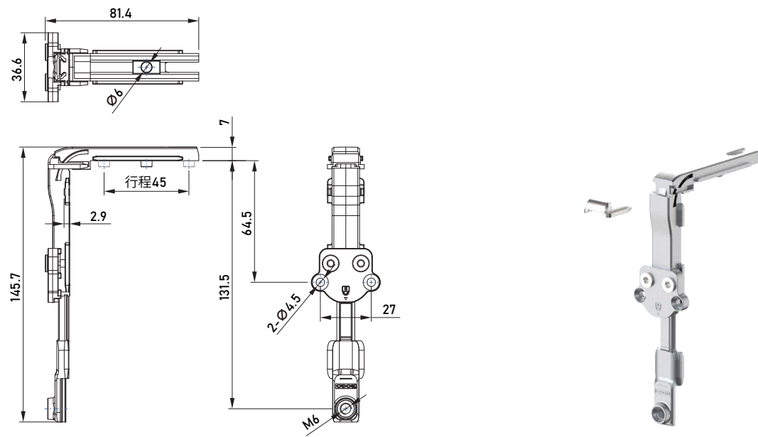
BG-SZJ03转角器 编号:F00097
