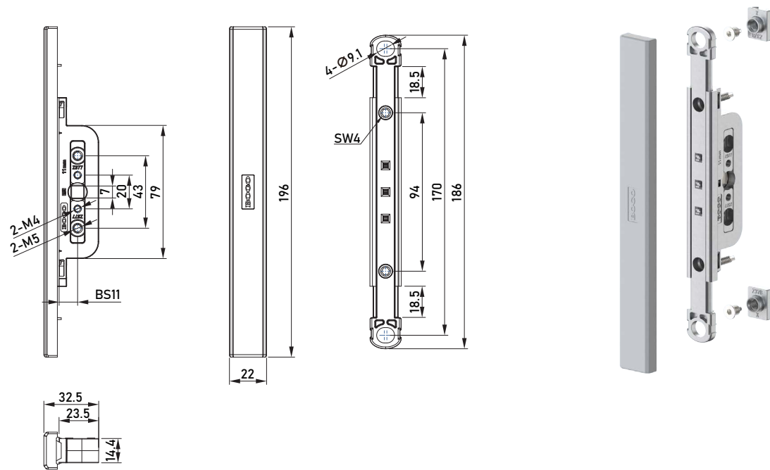
TQ11S单向传动盒 编号:G00060
